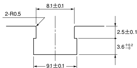
取付寸法図
